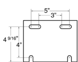
Mounting Plate (GBA-642, GBA-542)
