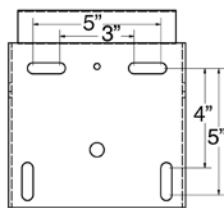
Mounting Plate (GBA-648, GBA-548)
