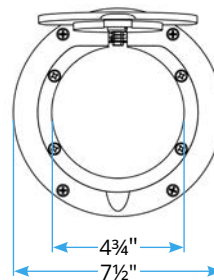
Standard PVB-711, PVB-75CVR-CP
